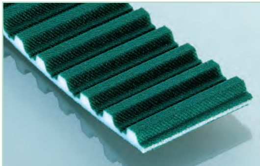
Cinghia con rivestimento sulla dentatura "PAZ"
